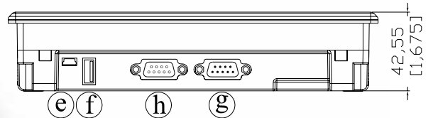
底視圖
