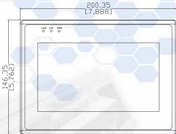
正視圖
