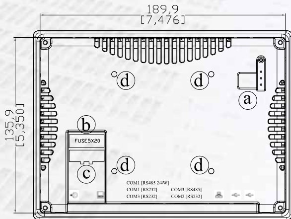
後視圖
